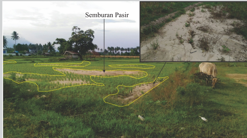
Contoh semburan pasir yang terjadi merata di area pesawahan daerah Lolu - Jonooge akibat gempa Palu 28 September 2018
