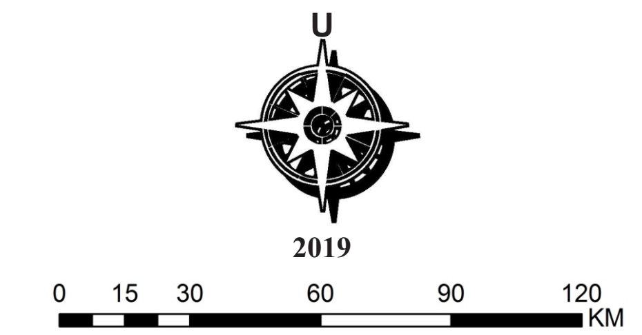
PETA ZONA KERENTANAN LIKUEFAKSI PROVINSI SULAWESI SELATAN
